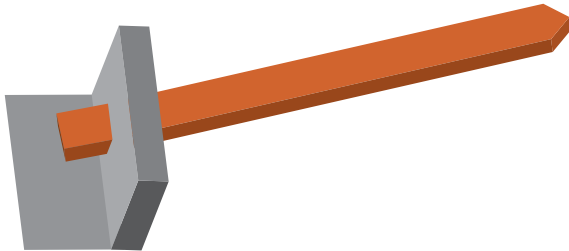
flusso di calore disperso - inverno parete standard in calcestruzzo
