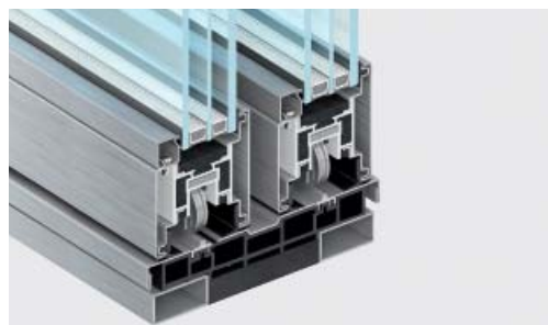
nodo inferiore con soglia integrata | h 97-122 mm
