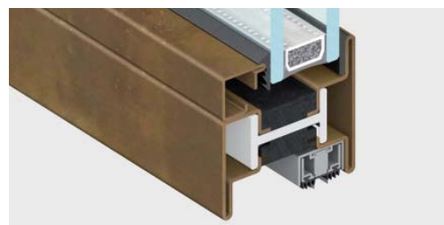
zoccolo | sezione in vista 54 mm
