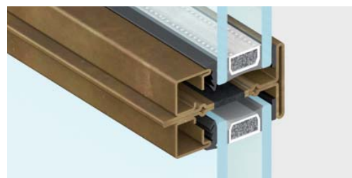
traverso dividi vetro | sezione in vista 36 mm
