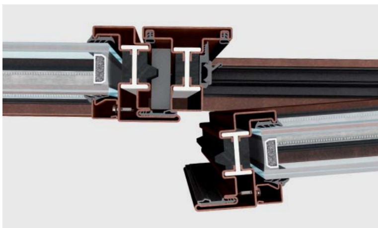
nodo centrale ridotto** | sezione in vista 85 mm
