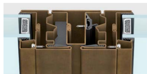
nodo centrale | sormonto | sezione in vista 145 mm
