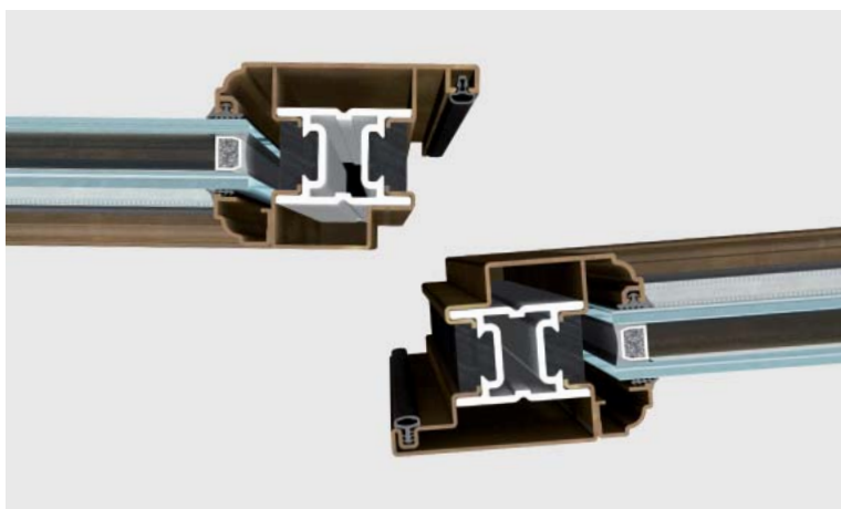
nodo centrale | sezione in vista 152 mm
